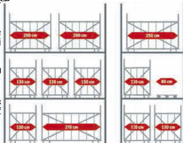
Regał na Corletty (szerokość mm, głębokość mm)
